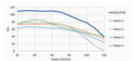
Drehmoment [Nm] an der Tretkurbel über Kadenz[U/min]
