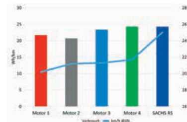
Geschwindigkeit [km/h] und Energieverbrauch bei einer Steigung von 6%
