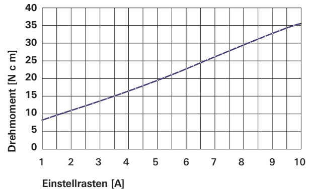
Drehmoment-Kennlinie
