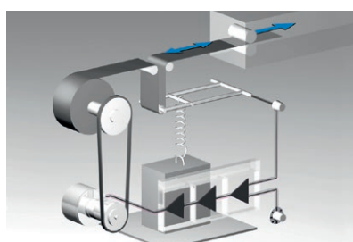
Geregelt Kraftregelung mit Tänzer
