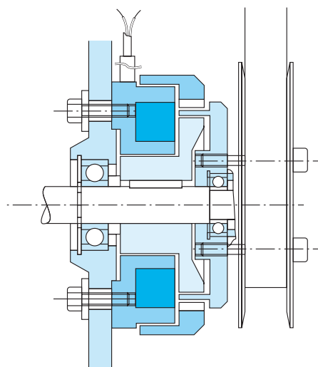
Hysteresiskupplung zum Aufwickeln von Folie mit konstanter Zugkraft.
