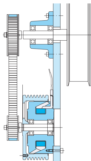
Hysteresisbremse zum Abwickeln eines Bandes mit konstanter Zugkraft. Um ein höheres Bremsmoment zu realisieren, wird hier eine Zahnriemenübersetzung eingesetzt.
