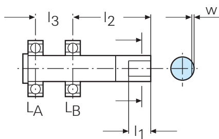
Anordnung Welle / Lager
